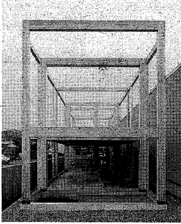
Sボルトによる耐力壁なしの木造住宅躯体
